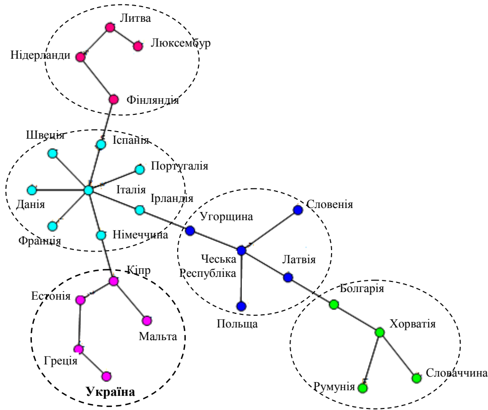
Рис. 4. Мінімальне остівне дерево (галузевий вигляд) для показника „Внесок туристичної галузі до ВВП”
